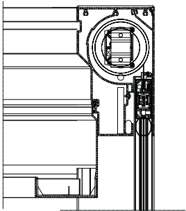
Brio Swing - Querschnitt
