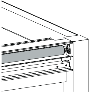
Aufwickelwelle im Balken integriert
