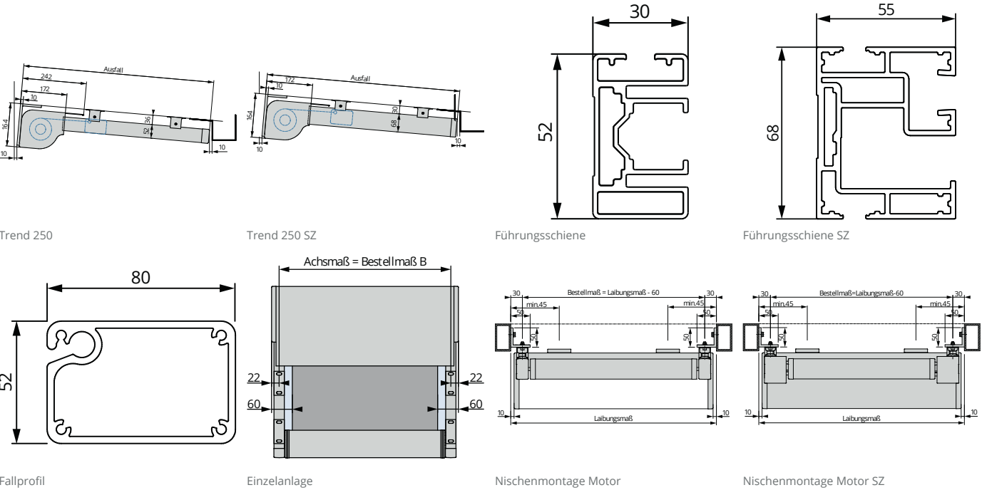
Fallprofil Einzelanlage Nischenmontage Motor Nischenmontage Motor SZ
