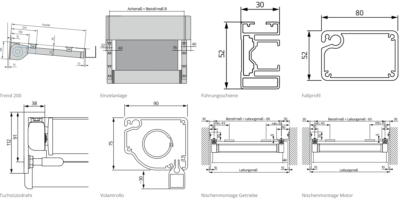
Trend 200 Einzelanlage Führungsschiene Fallprofil Tuchstützdraht Volantrollo Nischenmontage Getriebe Nischenmontage Motor
